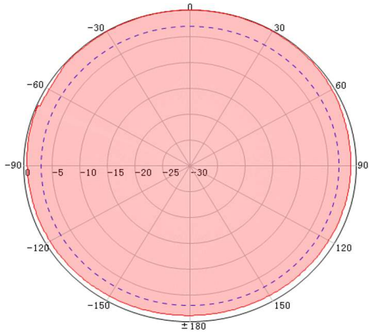
960MHz Horizontal
