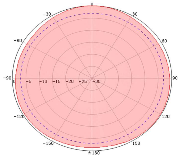
2100MHz Horizontal
