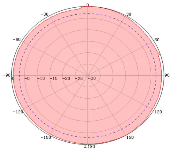
1800MHz Horizontal
