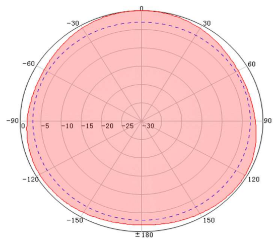
1800MHz Horizontal
