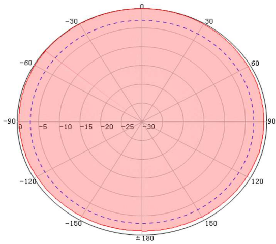
960MHz Horizontal
