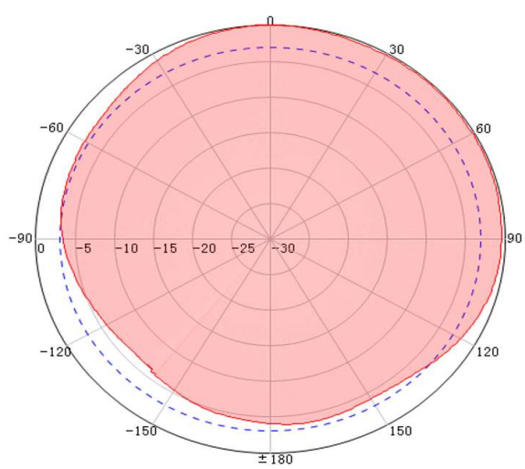
2600MHz Horizontal
