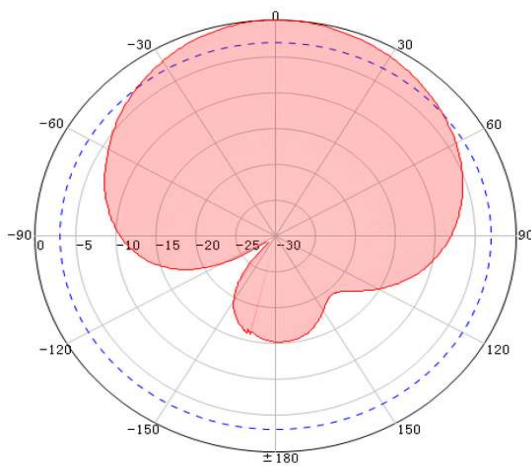
700MHz V Plane
