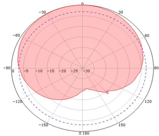
700MHz H Plane
